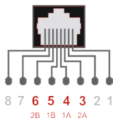
Kontakt-Belegung des ISDN-S 0 -Anschlusses
