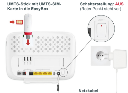
Netz Kabel
